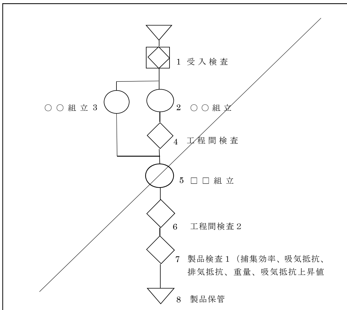
添付図9 製造工程のフローチャートの記載例 (全面改定)
