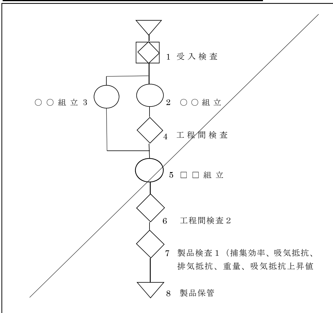
添付図9 製造工程のフローチャートの記載例 (全面改定)
